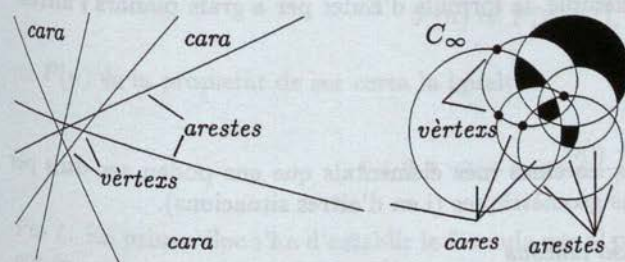
Figura 2. Disseccions amb vèrtexs, arestes, cares (algunes les hem indicat gràficament omplint-les de negre), algunes fitades i d'altres no; en el cas que hi hagi un única cara no fitada la indicarem per C_{\infty} .
